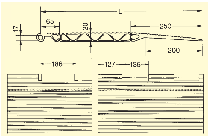
Versio 3:n liitännärakenne
